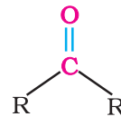
कीटोन
