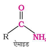
एमाइड
