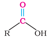
कार्बोक्सिलिक अम्ल
